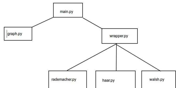
Рисунок 1 – Структура розробленого програмного пакету
