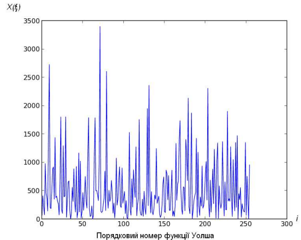
Рисунок 9 – Значення X(f_i) , які отримані при розкладі випадкової величини в спектр за функціями Уолша
